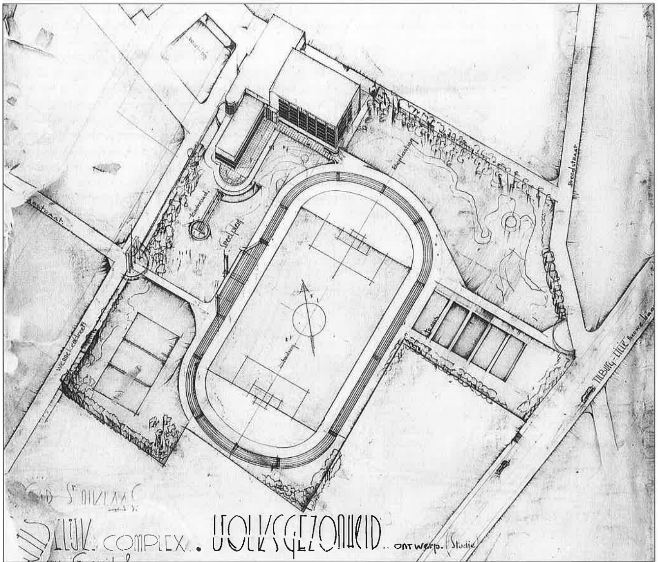
Grondplan van het stadion met zwembadinstallatie.
